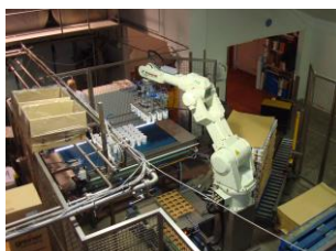
Kawasaki FS060L bij yoghurtfabriek bekers in trays zetten en palletiseren
