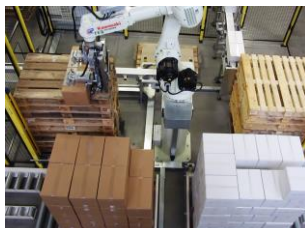
Kawasaki RD080N bij Ardeca Belgium dozen van 2 vullijnen palletiseren
