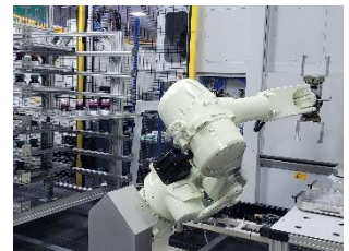
Kawasaki RS080N met RFA-JobEdit en ladekast bij Spinner freesmachine
