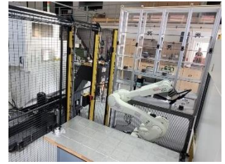
Kawasaki RS020N met RFA-Raster en RFA-Pallet bij Mazak freesmachine
